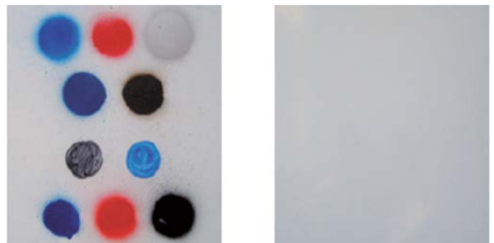
Przed i po 15 cyklach nakładania i usuwania graffiti
